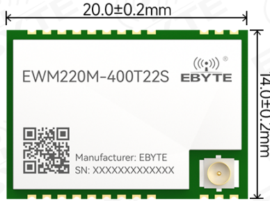
图 1: EWM220M-400T22S
