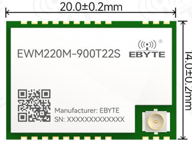
图 2: EWM220M-900T22S
