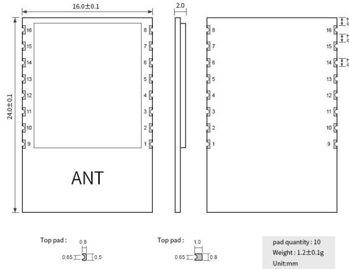
图 3-1 机械尺寸与引脚定义
