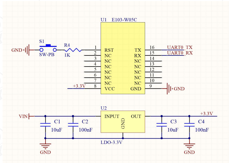
图 5-1 电路图
